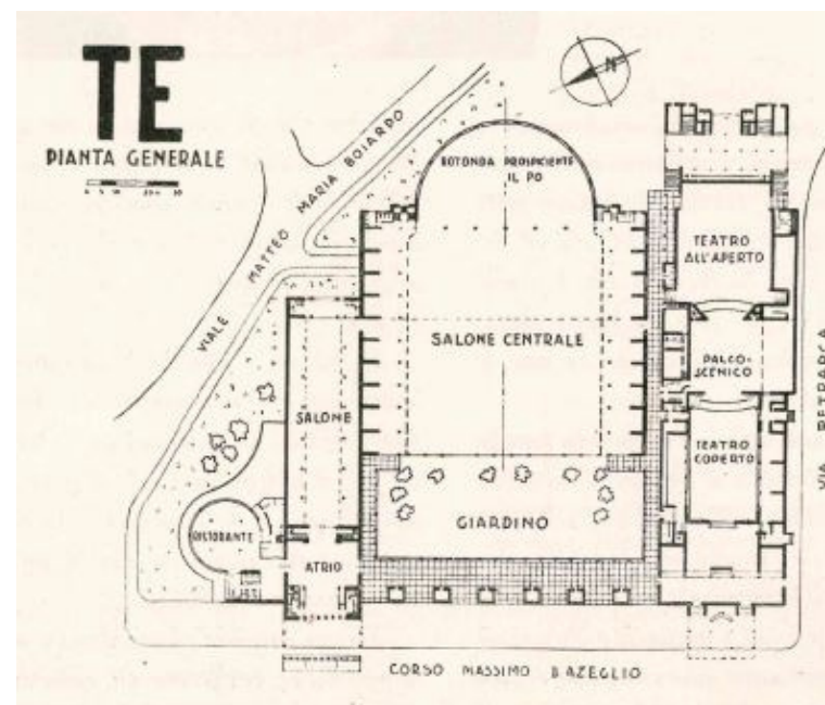
1948. Il nuovo padiglione centrale. Architetto Roberto Biscaretti di Ruffia e ingegner Pierluigi Nervi.
